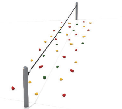
[ FUN-PECL07 ] 줄잡고 암벽오르기 식별번호 25041048 제품규격 5090×2000×3300 조달가격 6,050,000 원
